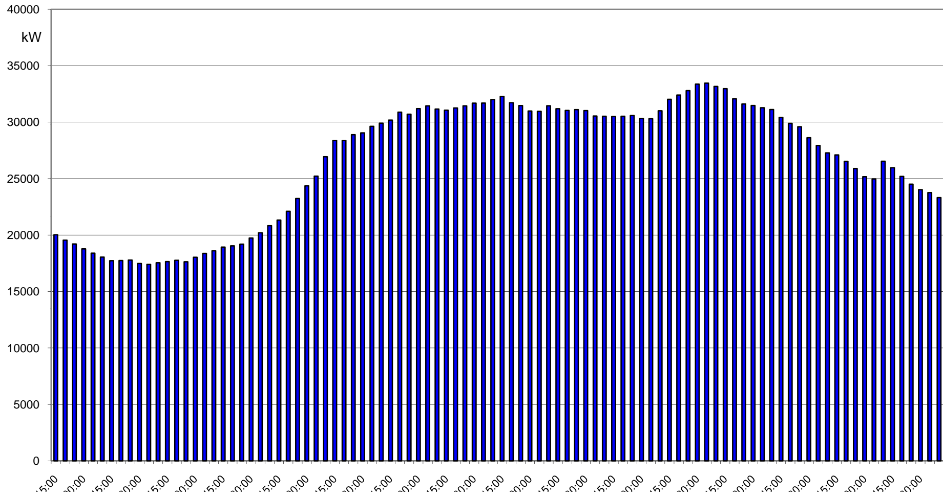
Lastverlauf des Jahreshöchstlasttages 03.12.2007
